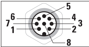
Disegno schematico connettore 12
