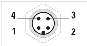
Schemazeichnung M12-Stecker
