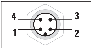
Schéma du connecteur M12
