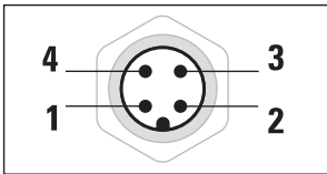
Disegno schematico connettore M12
