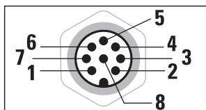
Diagrama del conector M12
