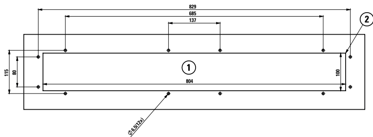
FIELDLED EVO 790_96 Einbau
