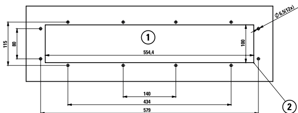
FIELDLED EVO 540_96 Einbau
