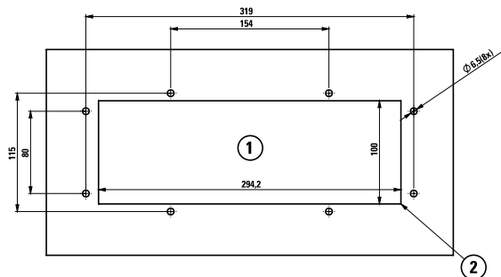
FIELDLED EVO 280_96 Einbau
