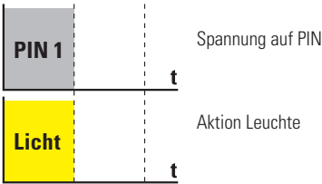
Mögliche Varianten M12-Stecker
