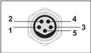
Schéma du connecteur M8
