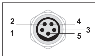
Disegno schematico connettore M8
