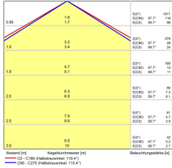
Abstand [m] Kegelhalbwinkel [°] Beleuchtungsstärke [lx] - - - C90 (Photobezweck 118.4°) - - - C80 (Photobezweck 115.4°)
